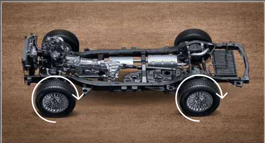
Electric Differential Lock – Front and Rear ระบบล็อกเฟืองขับเคลื่อนไฟฟ้าด้านหน้าและด้านหลัง
